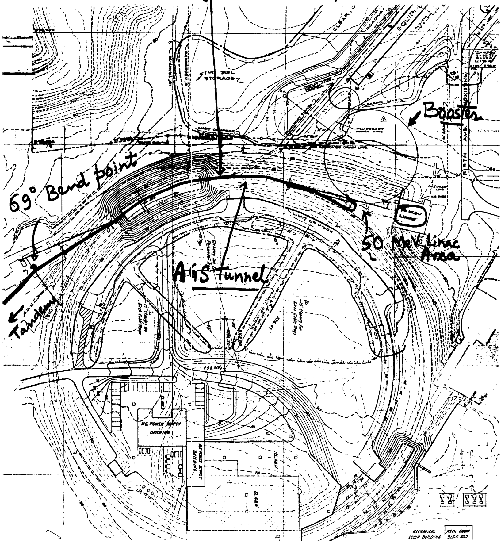
FIG 1. SITE PLAN
