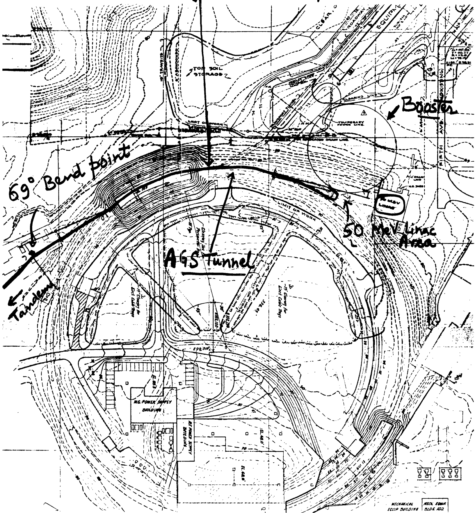
FIG 1. SITE PLAN
