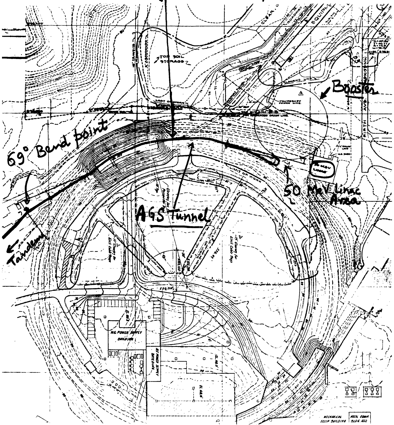
FIG 1. SITE PLAN
